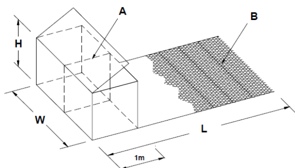
Obr.1 A Terramesh Systém
