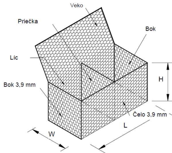
Obr.2 GABION SF so spevnenou čelnou a bočnou stenou so siete 3,9 mm (rôzne možnosti kombinácie podľa projektu)
