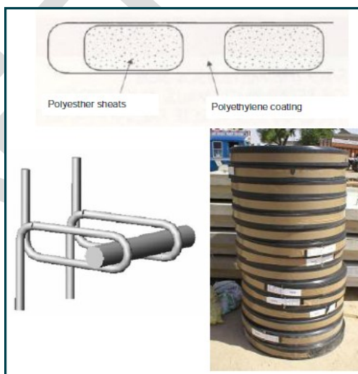
Systém Paraweb výstuže
